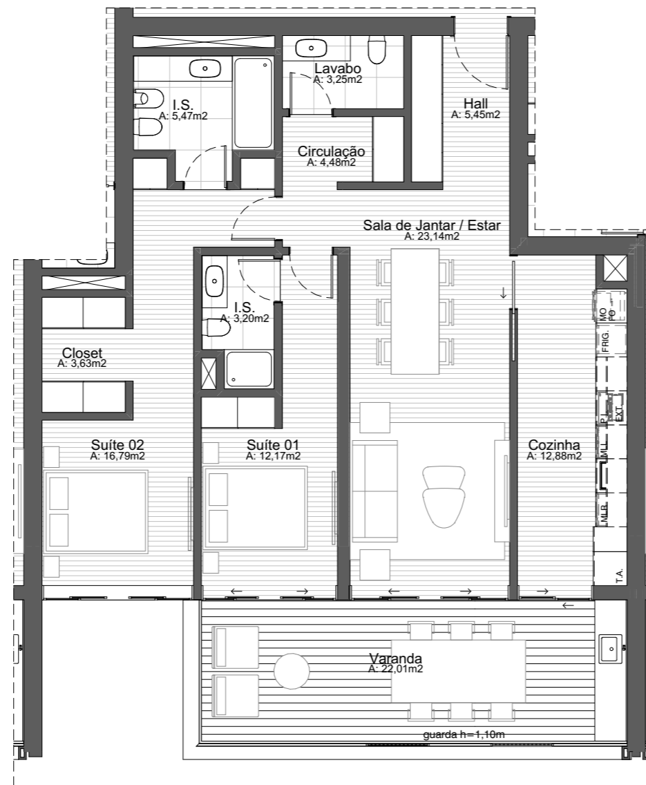
PLANTA - APARTAMENTO 4B 1:100
