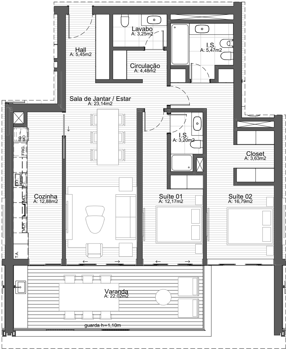
PLANTA - APARTAMENTO 4E 1:100
