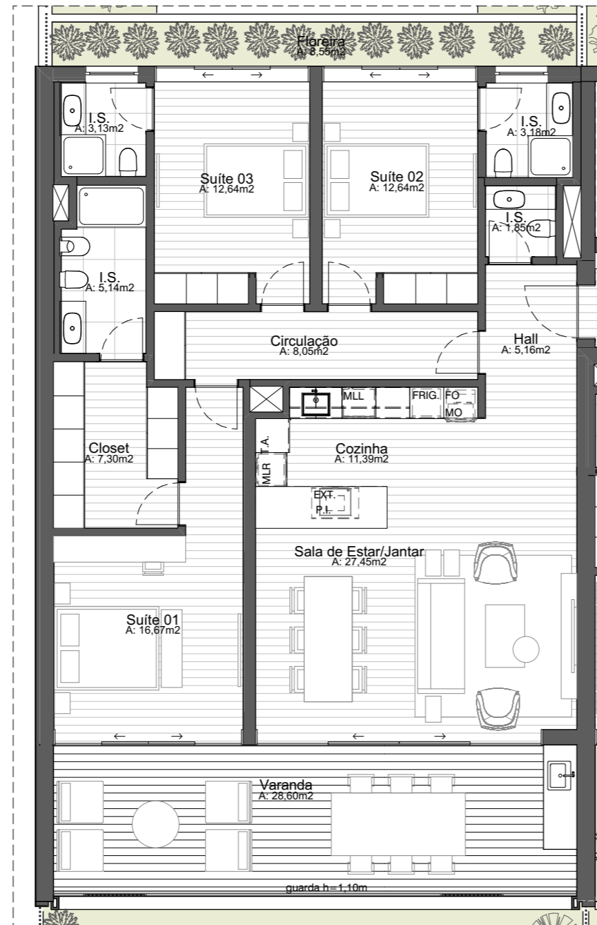
PLANTA - APARTAMENTO 0H 1:100
