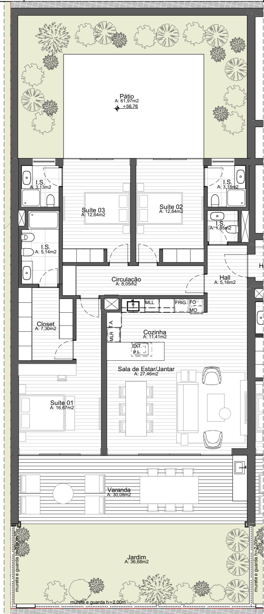
PLANTA - APARTAMENTO GARDEN H 1:100
