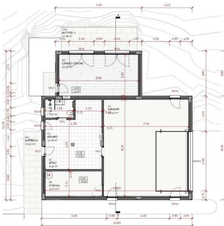
Planta Piso 0 Situação Definitiva
