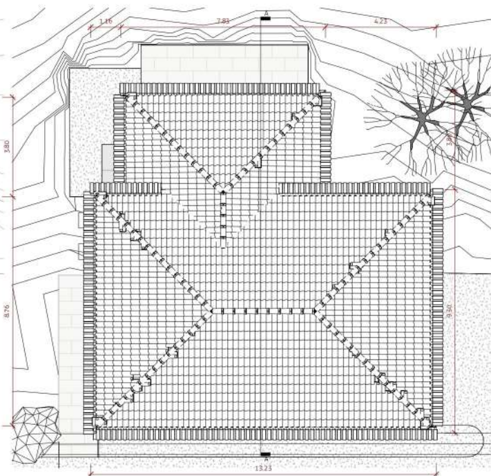
Planta de Cobertura - Situação Definitiva
